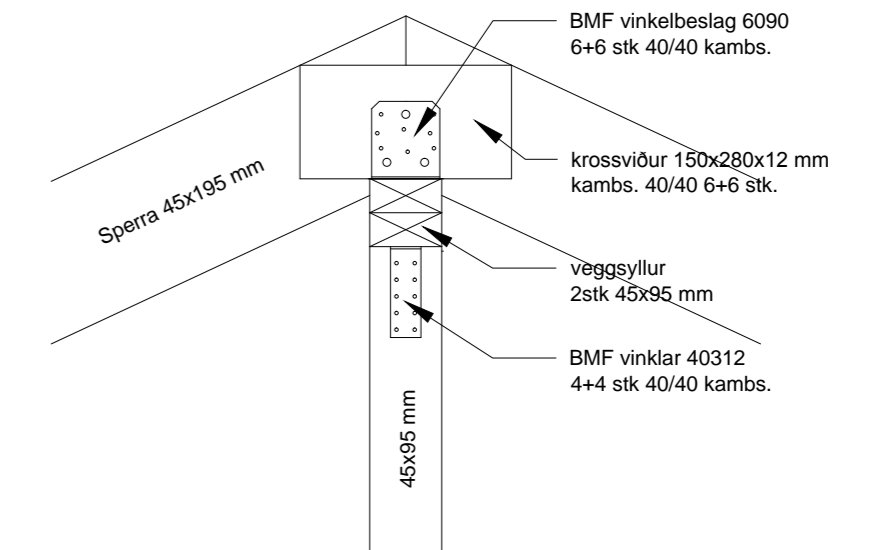
SNIÐ N-N (gestahús) sperrur á burðarvegg í mæni
