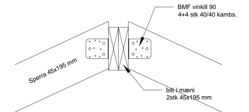
SNIÐ O-O (gestahús) sperrur og biti í mæni
