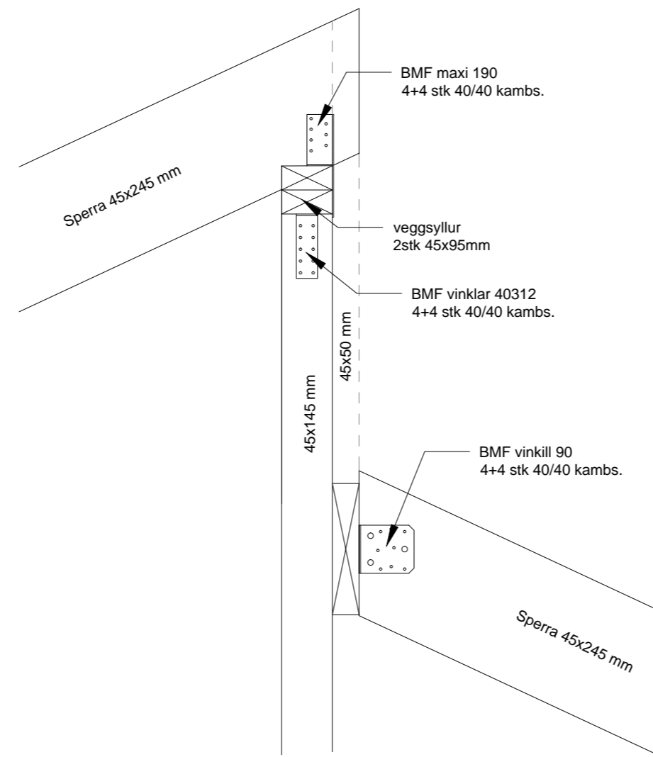
SNIÐ J-J (aðalhús) sperrur og milliveggur við mæni
