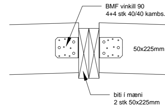
SNIÐ G-G sperrur millibygging
