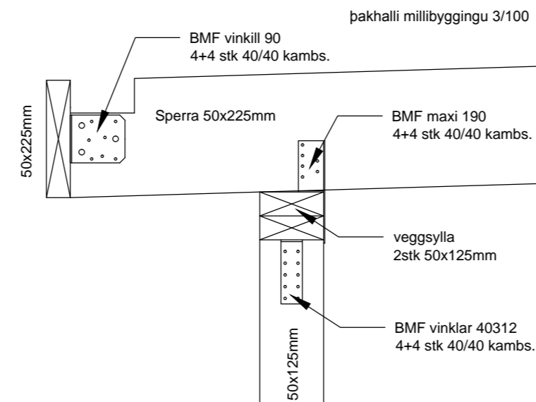
SNIÐ F-F sperrur millibygging
