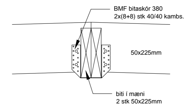
SNIÐ H-H biti millibygging
